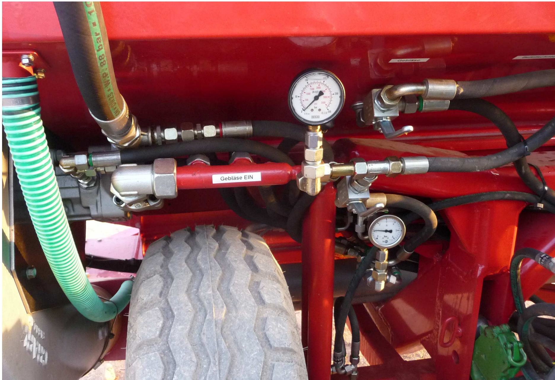
Frontdrucktank FDT2940K mit Kettendosierung Verteilersystem mit 2 Verteilern
