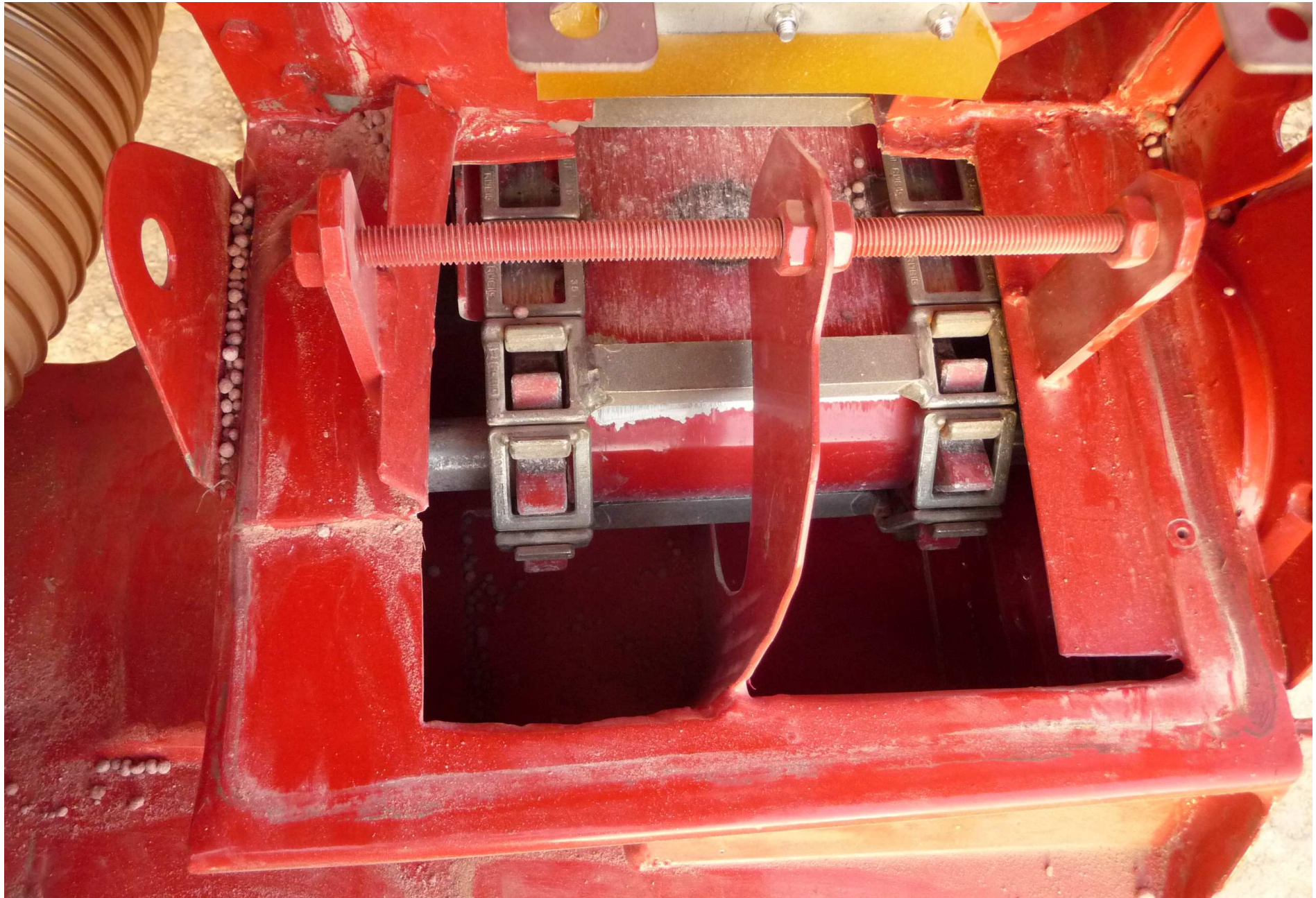
Frontdrucktank FDT2940K mit Kettendosierung Verteilersystem mit 2 Verteilern
