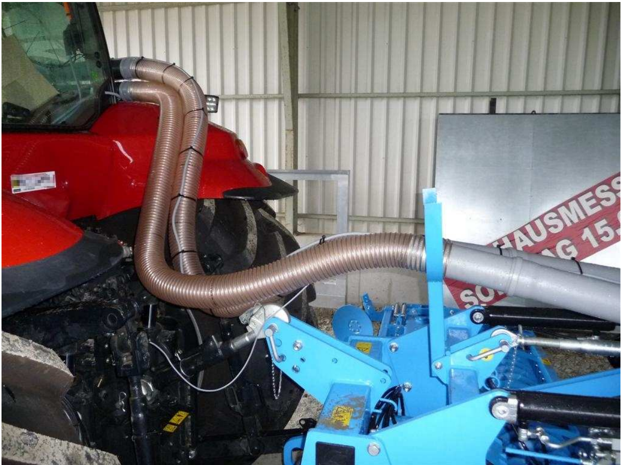
2 Förderleitungen Ø110 mm auf Lemken Säkombination, 6 m Arbeitsbreite - mit U-Halterung, auf Lemken Kreiselegge
