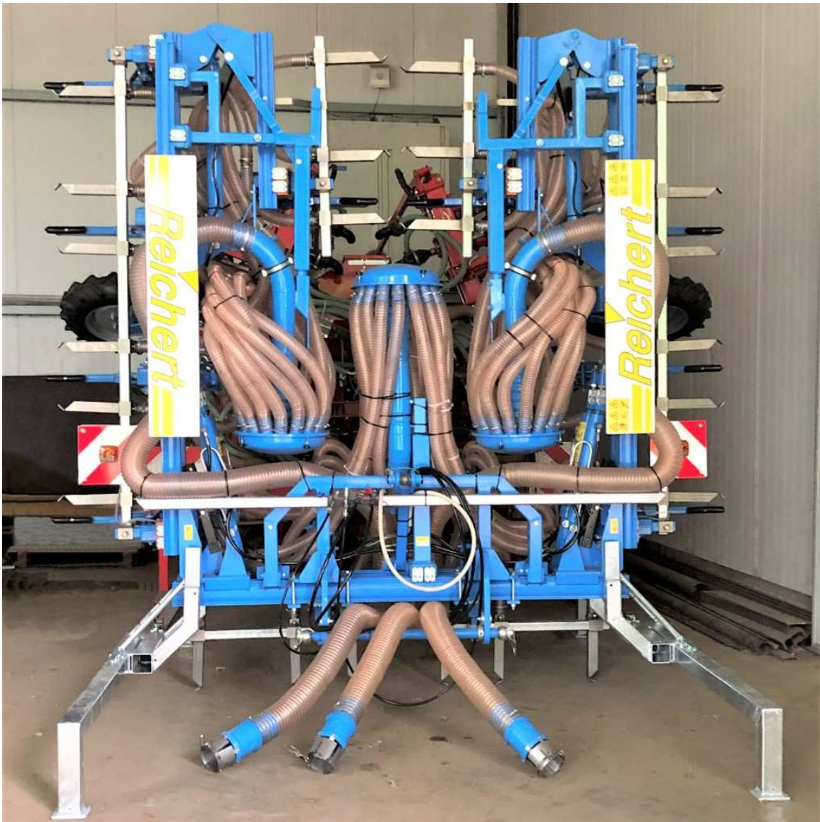
Heckdüngerahmen HDR 9/12, hydraulisch 4-fach geklappt 9 m Arbeitsbreite, 12 Reihen - mit Umschaltung: Unterfußdüngung in der Reihe oder seitliche Reihendüngung - mit Abstellstützen für sicheren Stand
